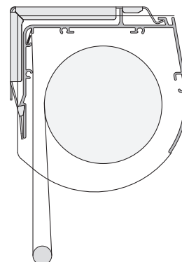
montage semikassett
