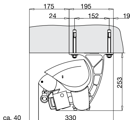
Takmontage
