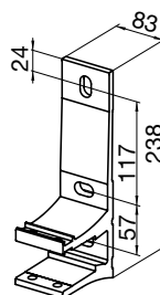
Väggkonsol
