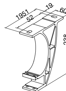
Takkonsol
